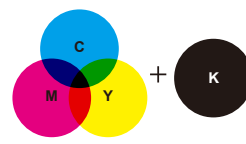
減法混色
